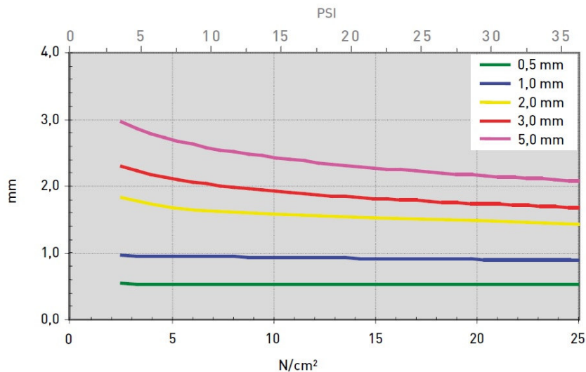
Druckabhängigkeit der Materialstärke bei CMC 15023
