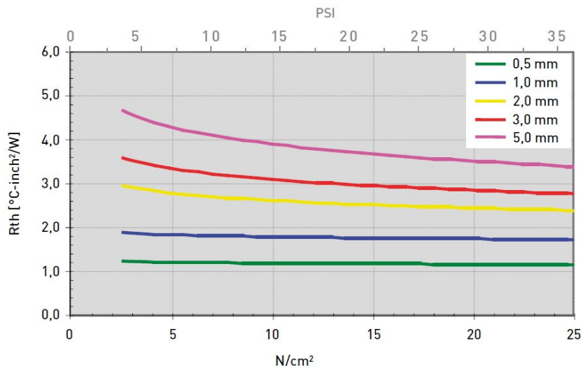
Druckabhängigkeit des thermischen Widerstands R_{th} bei CMC 15023
